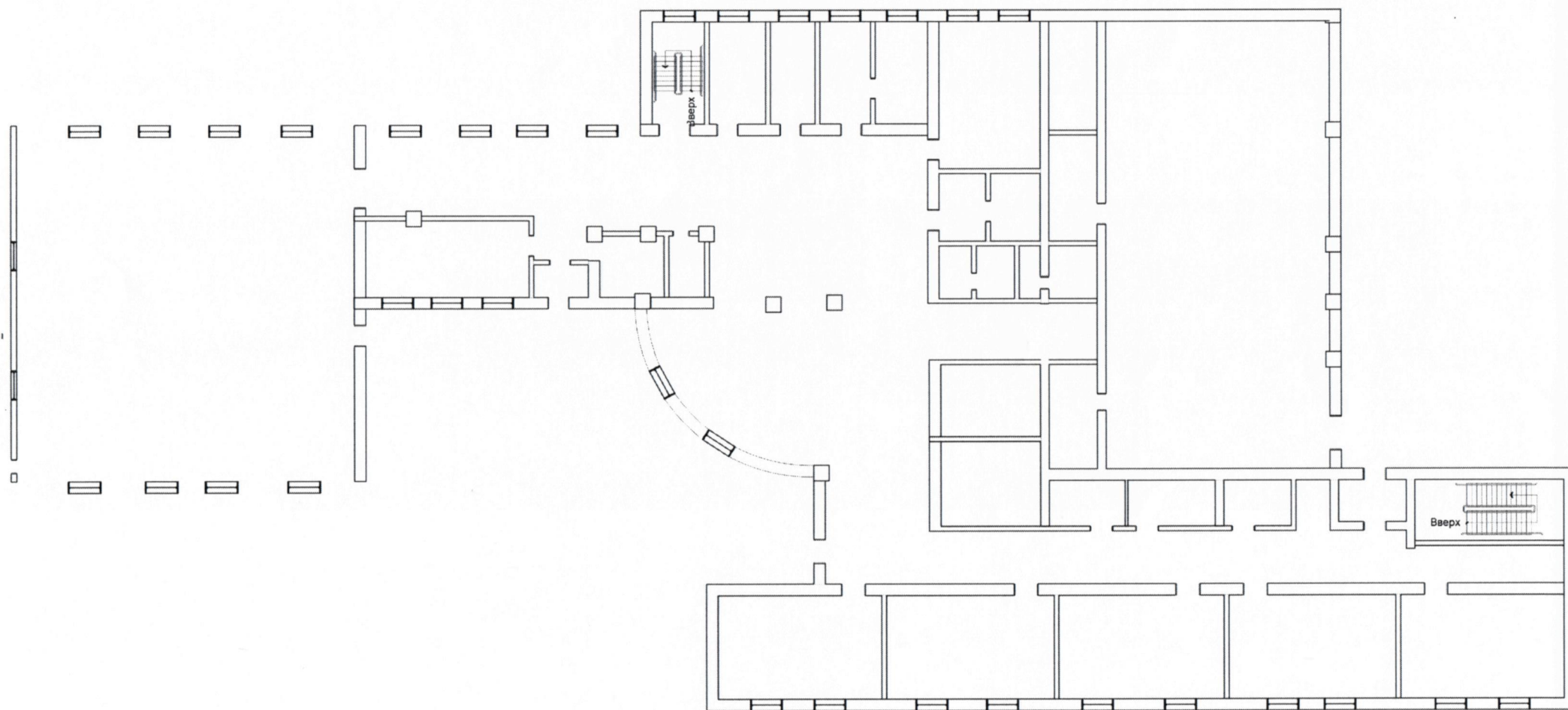
План 1 этажа
